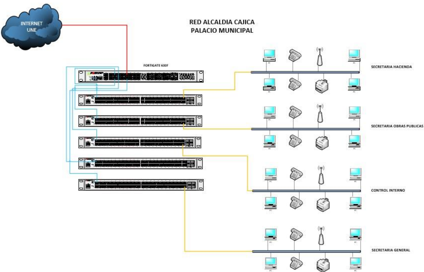
Figura 7 arquitectura networking imagen propia
