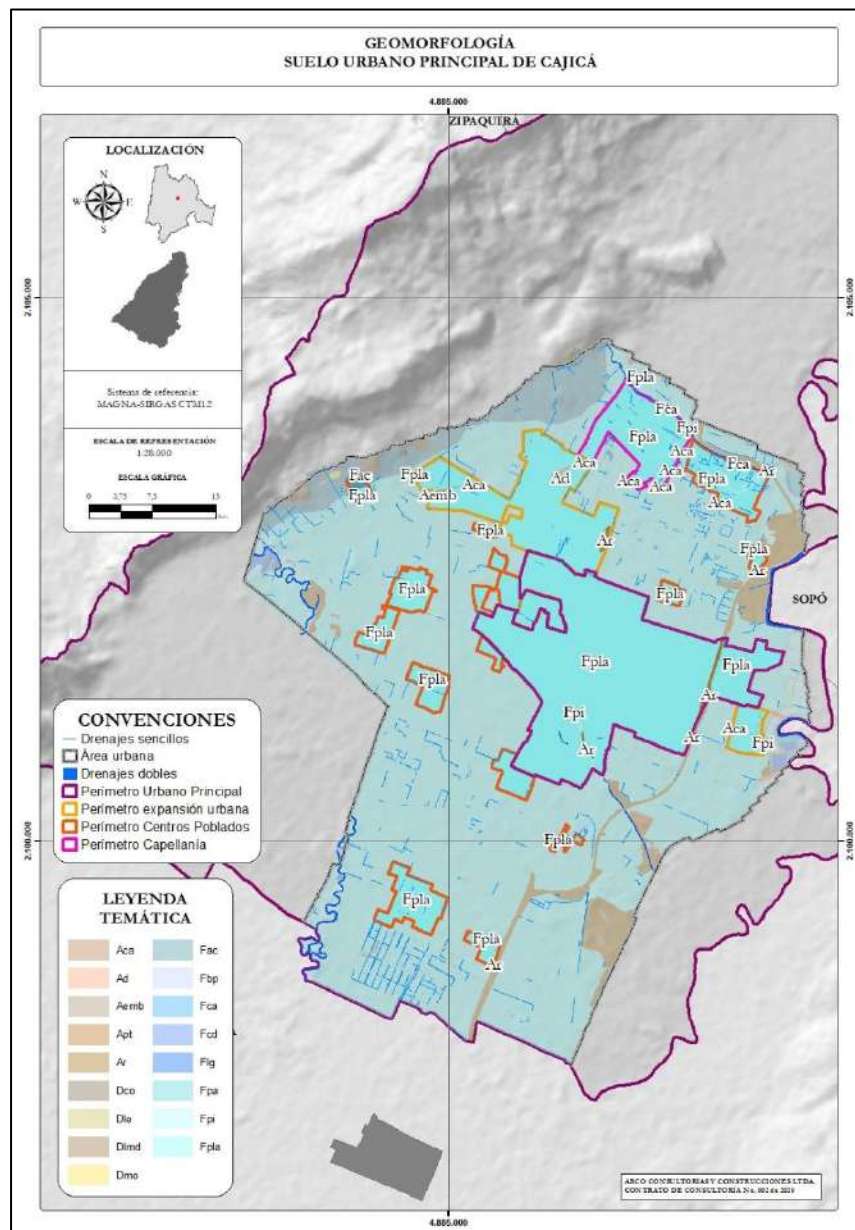
Ilustración 2. Geomorfología del suelo urbano principal, municipio de Cajicá. Fuente: Arco Consultorías y Construcciones Ltda. (2021).
