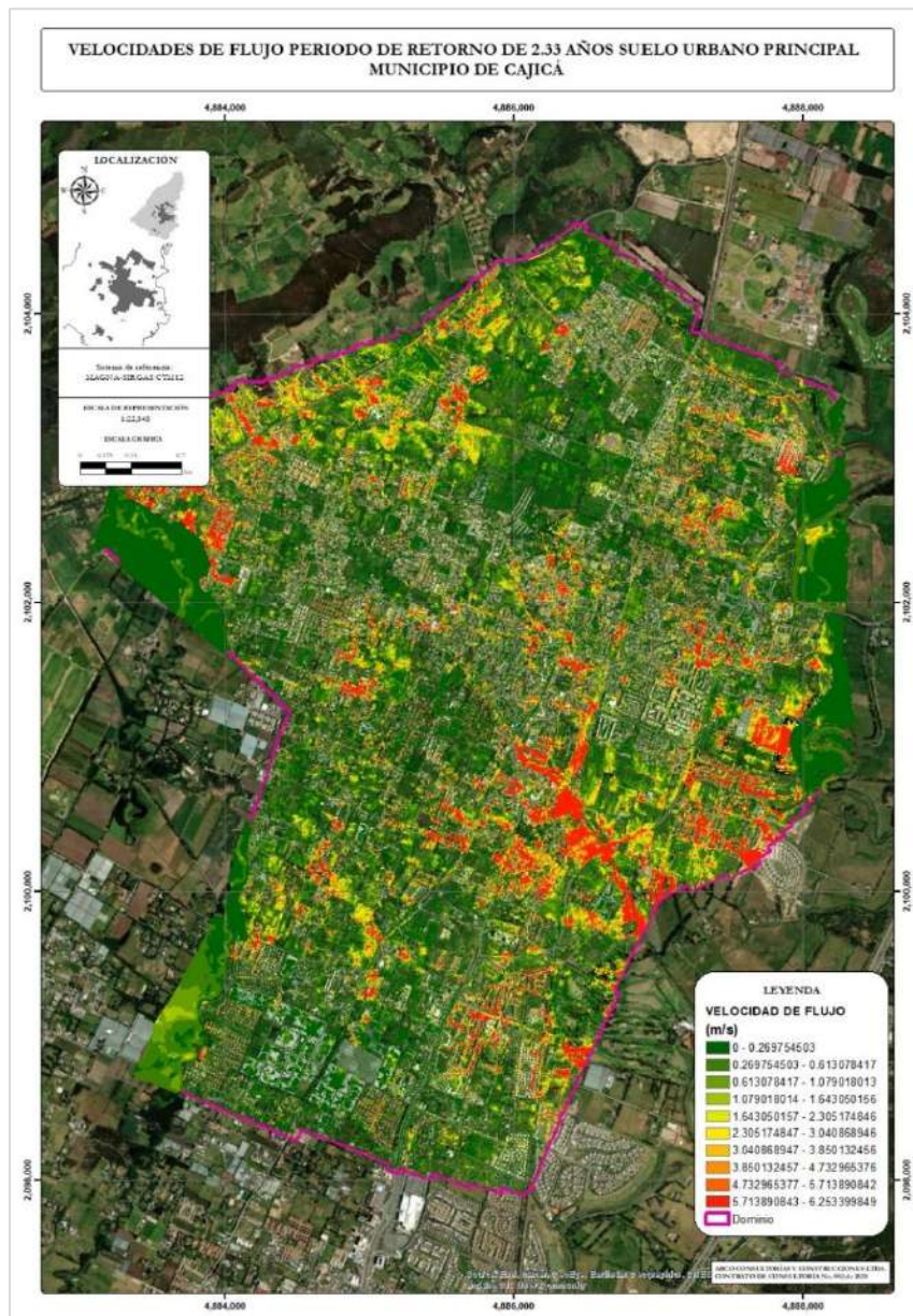
Ilustración 18 Resultados velocidades de flujo ( T_r=2.33 años) casco urbano de Cajicá. Fuente: Arco Consultorías y Construcciones Ltda. (2021)
