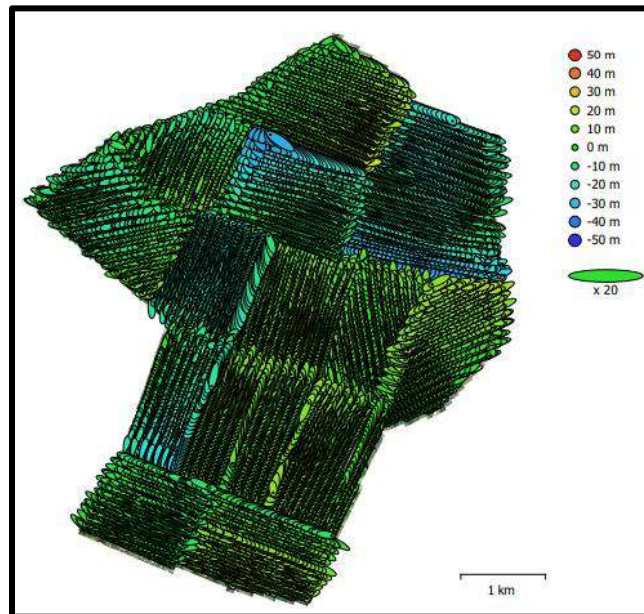
Ilustración 5. Ubicación de la cámara para las imágenes capturadas y altura promedio. Fuente: Agisoft Photoscan
