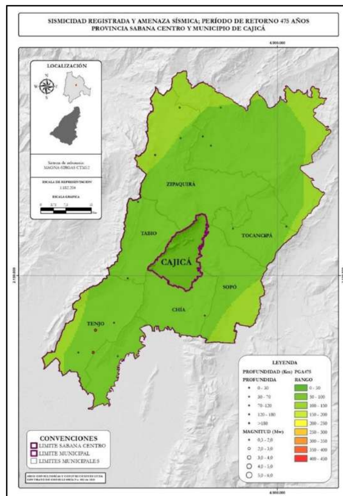
Ilustración 74. Sismicidad registrada y amenaza sísmica con período de retorno 475 años en el municipio de Cajicá, Cundinamarca.
