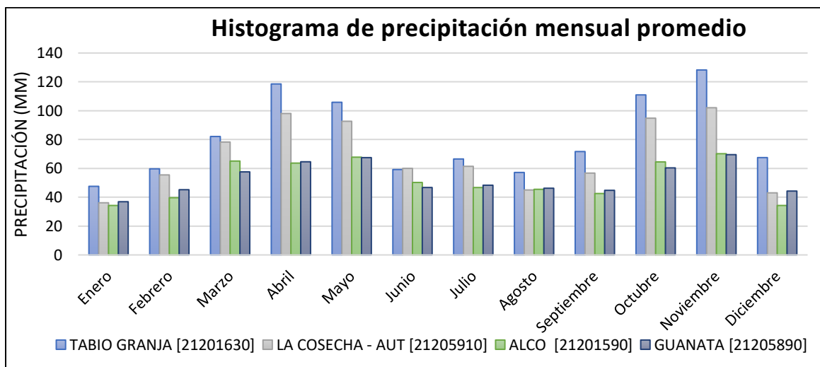
Ilustración 76. Histograma de precipitación mensual histórica de las estaciones evaluadas
