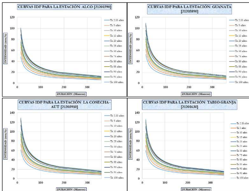
Ilustración 78. Mosaico de Curvas de Intensidad, Duración y Frecuencia (IDF) para las estaciones de análisis
