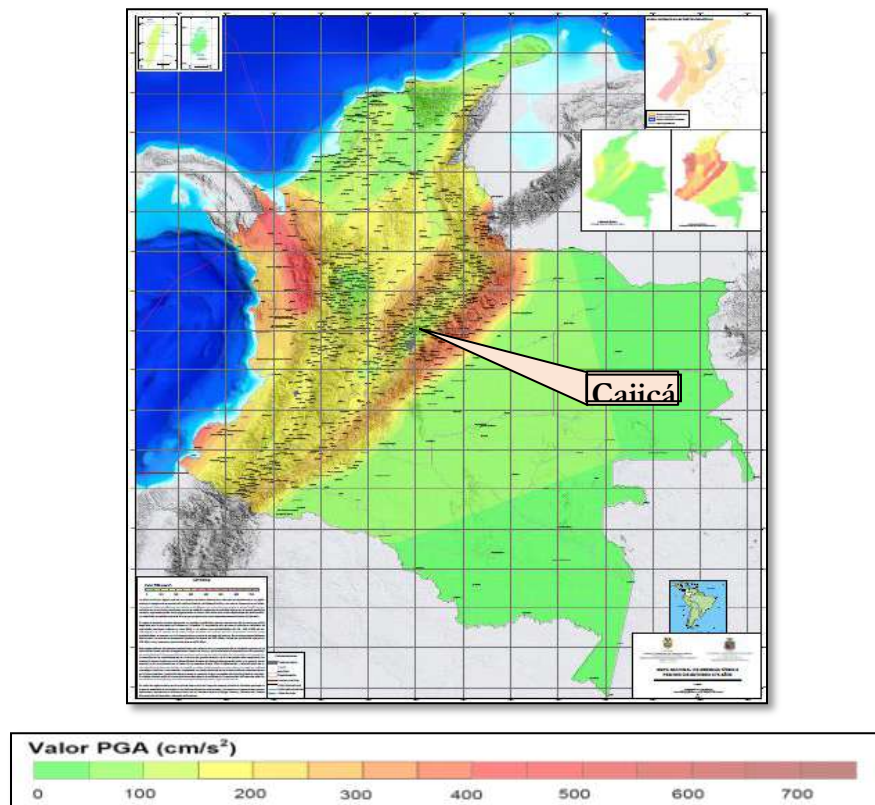
Ilustración 72. Zonificación sísmica para un período de retorno de 475 años.
