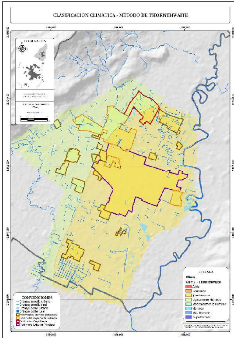
Ilustración 82. Clasificación climática por el método de Thornthwaite Fuente: Arco C&C, 2021
