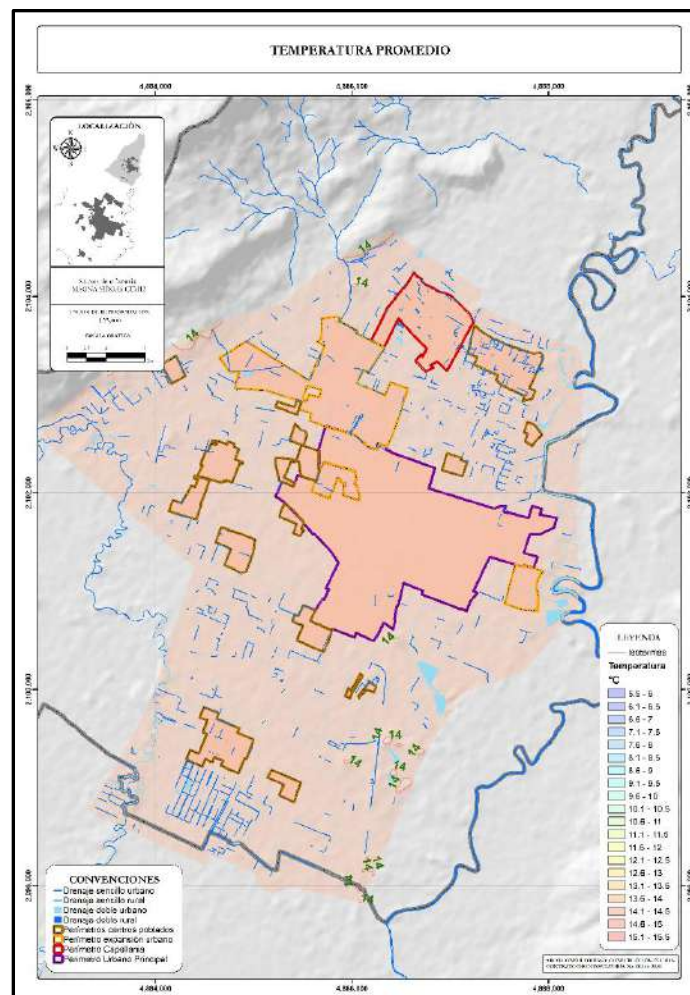
Ilustración 81. Temperatura anual multianual promedio Fuente: Arco C&C, 2021
