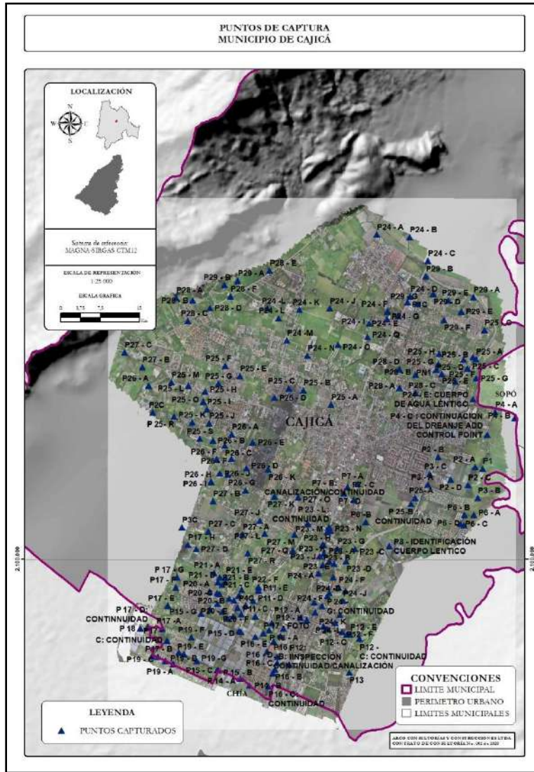
Ilustración 16. Puntos de captura de drenaje.
