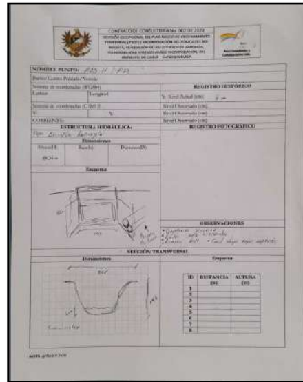
Ilustración 14. Formato estructuras hidráulicas.
