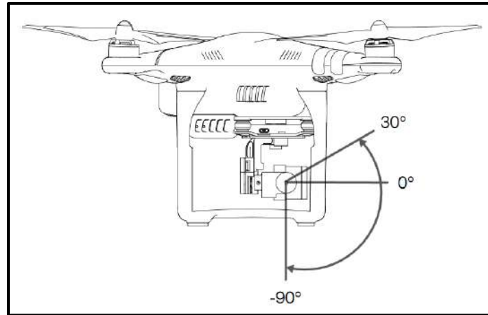
Ilustración 3. Ángulos de captura Gimbal, Phantom 4 Professional
