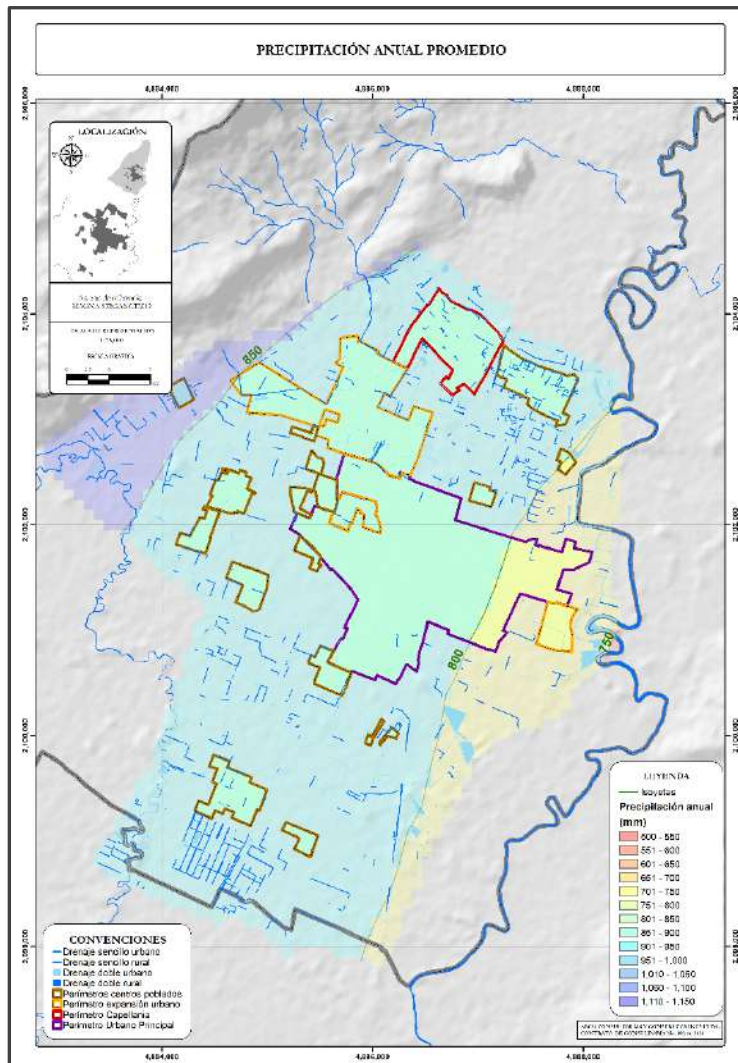
Ilustración 77. Precipitación anual promedio
