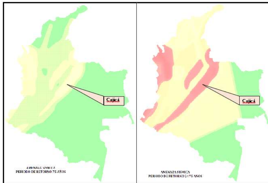
Ilustración 71. Mapa de sismicidad para períodos de retorno de 75 años (izq.) y 2475 años. Fuente: Servicio Geológico Colombiano (2016).
