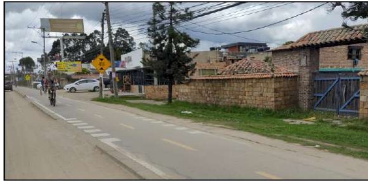
Ilustración 70. Planos y campos de llenos antrópicos. Fuente: Arco Consultorías y Construcciones Ltda. (2021).
