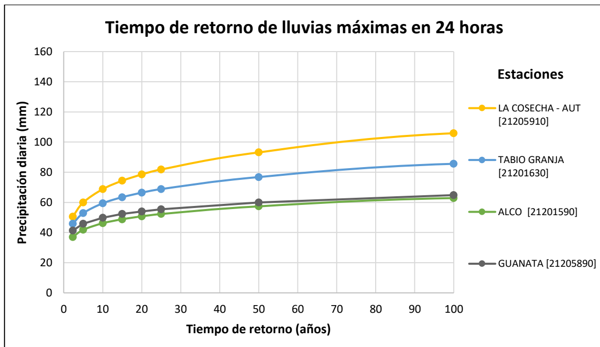
Ilustración 79. Lluvias máximas para periodos de retorno de 2.33 a 100 años. Fuente: Arco C&C, 2021
