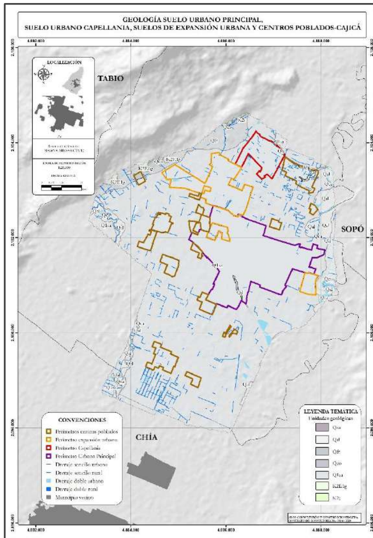
Ilustración 50. Mapa geológico del Suelo urbano principal, suelo urbano capellanía, suelos de expansión urbana y centros poblados.
